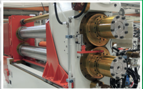
BLOCCAGGIO LAME AUTOMATICO AUTOMATIC BLADES LOCKING
